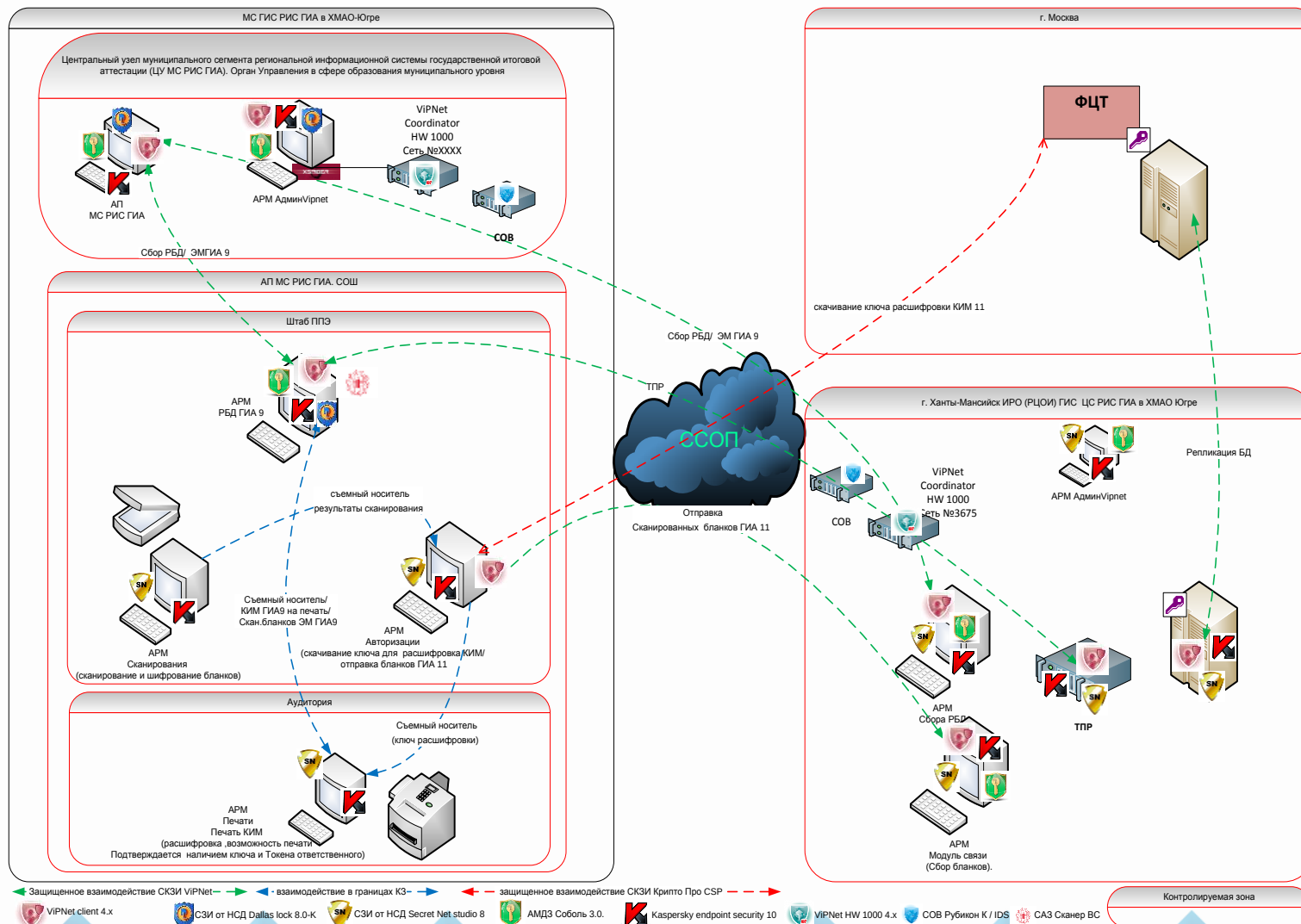
Принципиальная схема функционирования РИС ГИА в ХМАО - Югре
